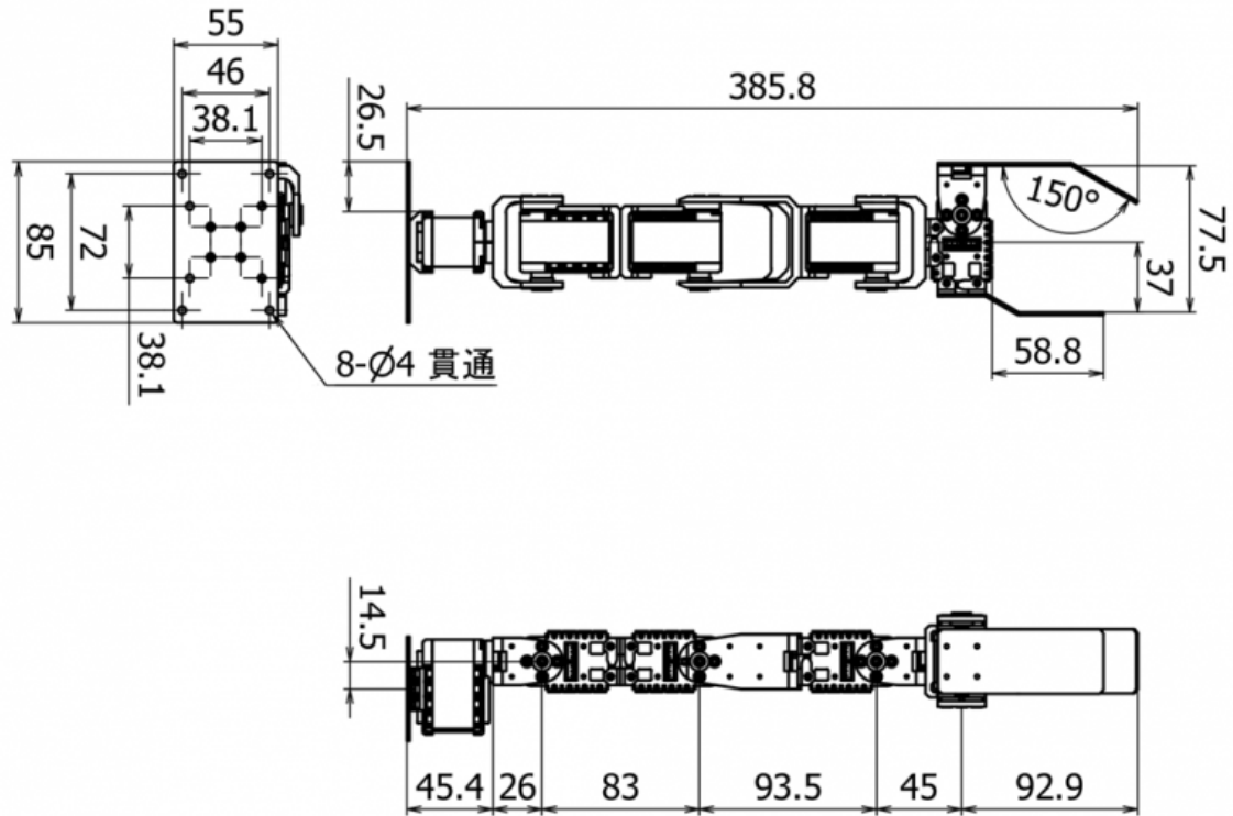
CRANE+ V2 寸法図
